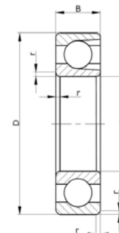
170 000 (200; 300; 400)
