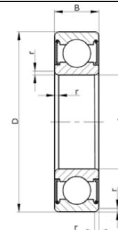
80 000 (6000 ZZ)
