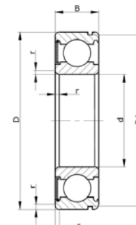
150 000 (6000 NZ)
