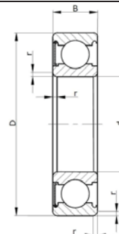
60 000 (6000 Z)
