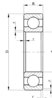
710 000 (6000 V)
