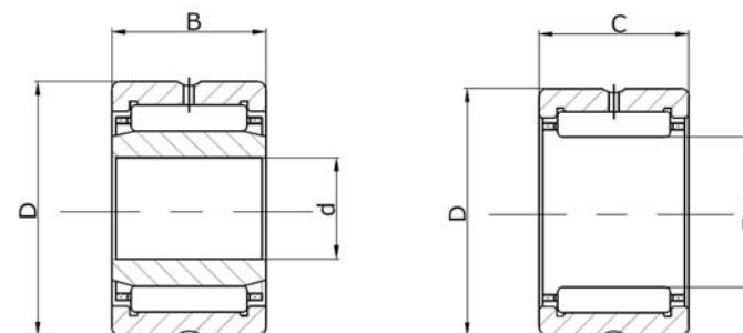
244... (NA 4...)
