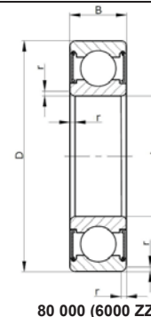
80 000 (6000 ZZ)
