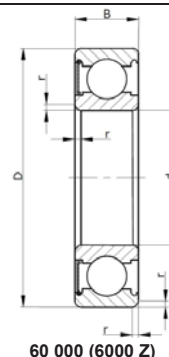
60 000 (6000 Z)
