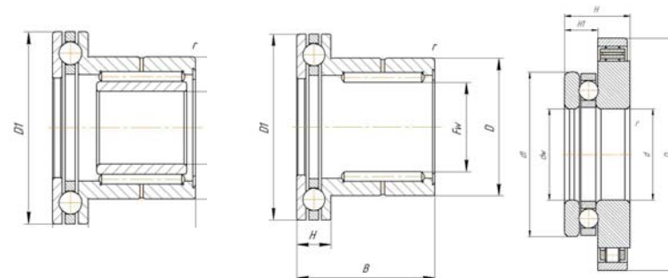
484 000 (NKXR...+IR)
