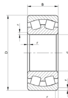
3 000 (2....CA; CAC)
