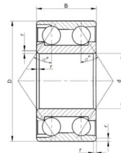
3 056 000 (3000 A)
