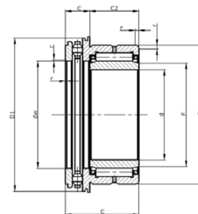
594 000 (NKXR...+IR)
