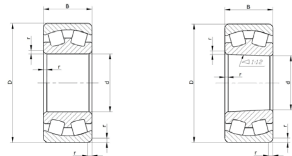
3 000 (2....CA; CAC)
